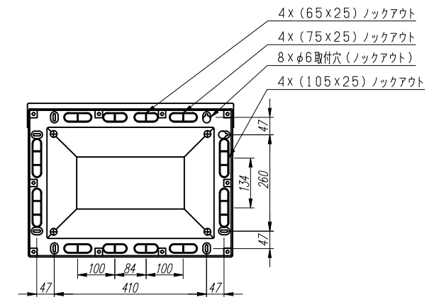
ボックス裏面図
