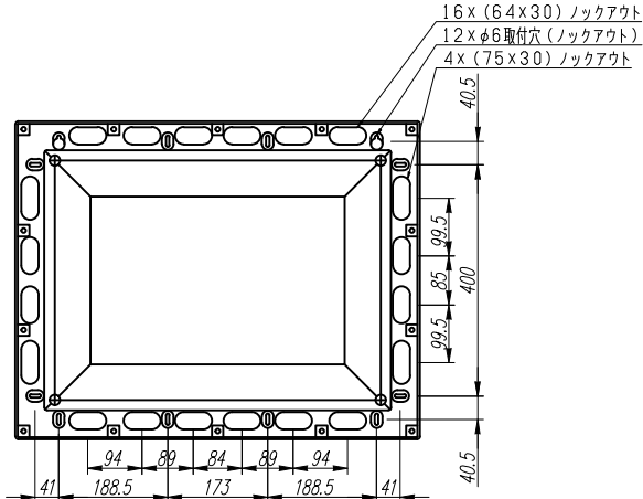
ボックス裏面図
