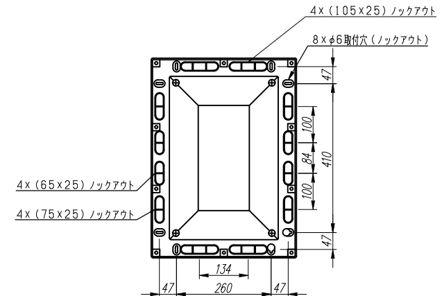
ボックス裏面図
