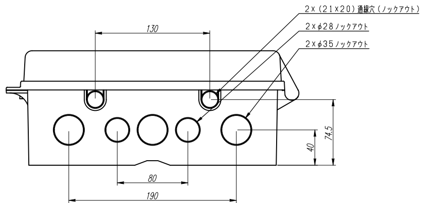
Y部断面 (1/1)
