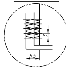
Y部断面 (1/1)
