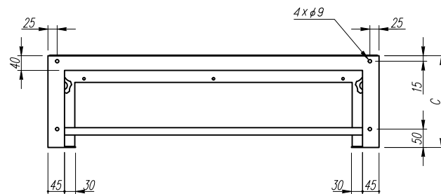
下面図
