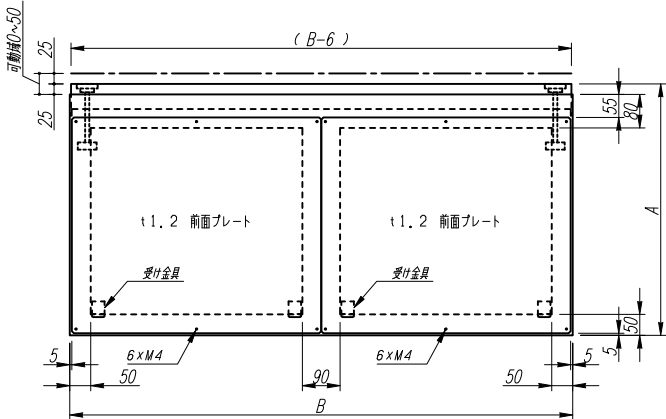
正面図
