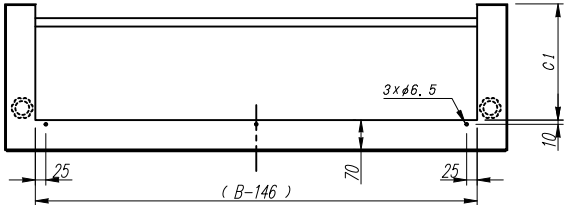
上面図
