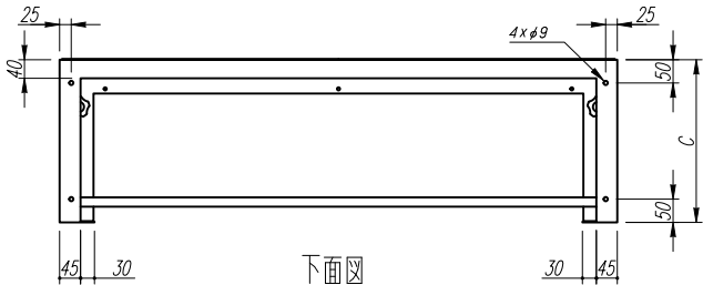
下面図
