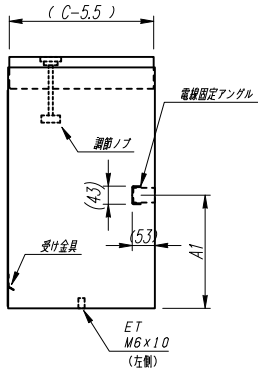
側面図
