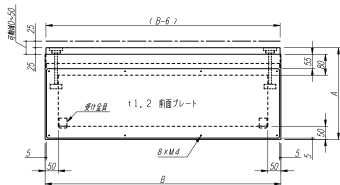
正面图
