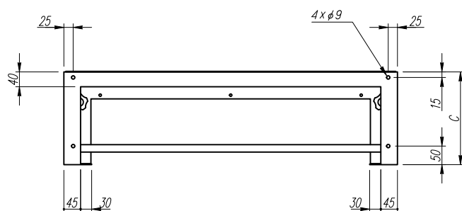
下面图
