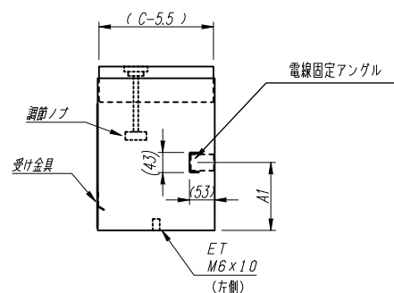
側面図
