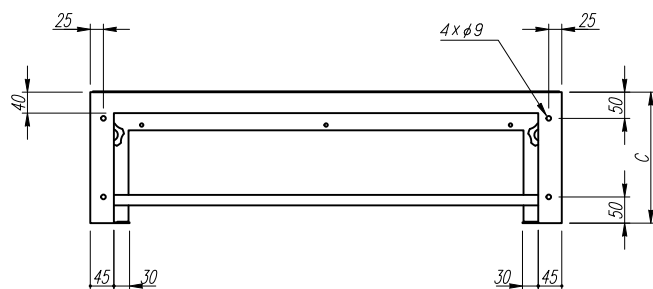
下面圖
