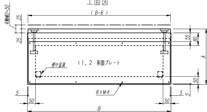
正面図
