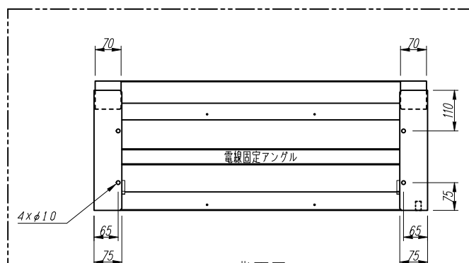
背面図
