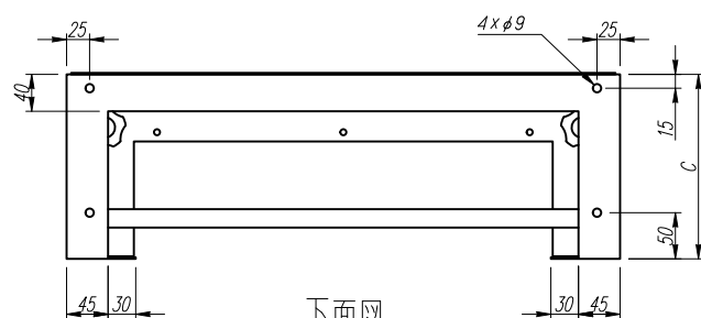
下面义
