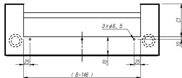
上面図
