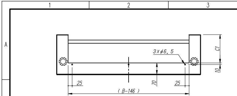
上面図
