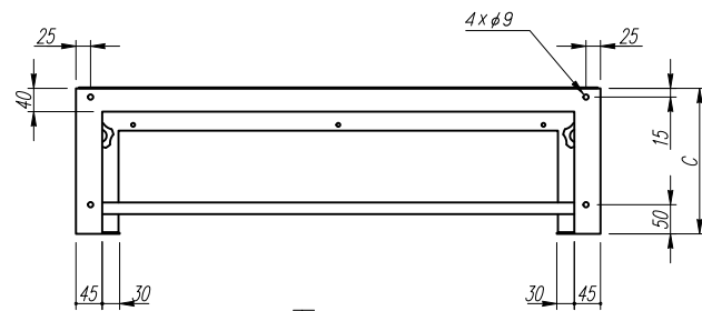
下面図
