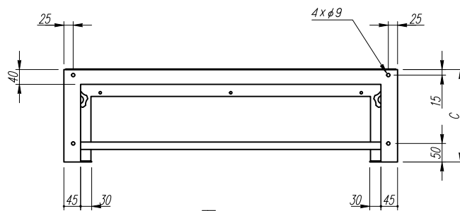
下面図
