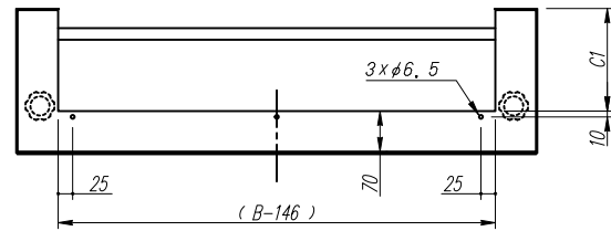
上面図
