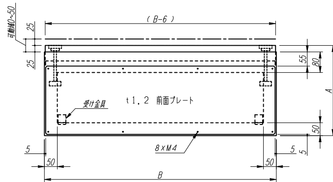
正面図
