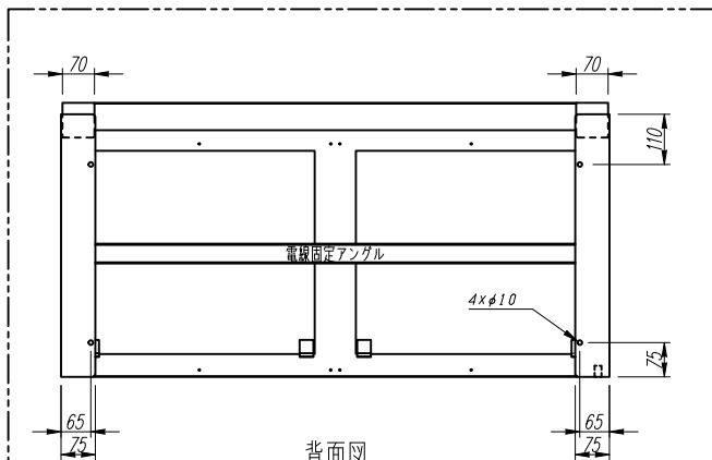
背面図
