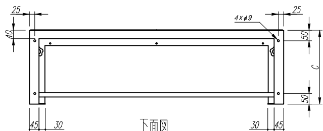
下面図
