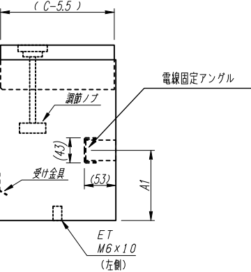
側面図
