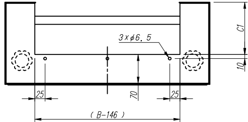
上面図
