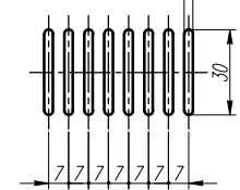
スリット部詳細図 (縮尺 1/2) 3
