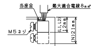
主幹用漏電遮断器端子構造
