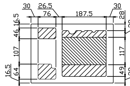
配線孔寸法図(//部開口, \\\部分岐背面)
