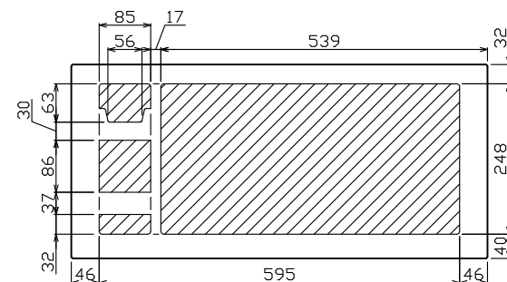
配線孔寸法図&lt;///部開口&gt;
