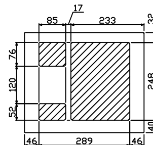
配線孔寸法図(ノックアウト)
