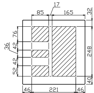
配線孔寸法図(断開口)
