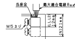
主幹用漏電遮断器端子構造
