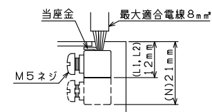
主幹用漏電遮断器端子構造
