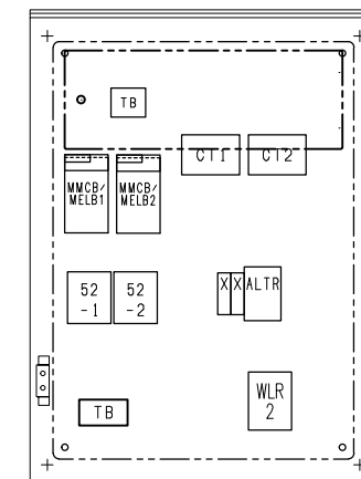
パネル裏面配置図
