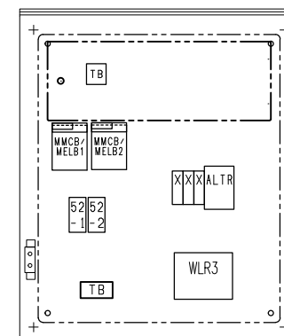
パネル裏面配置図
