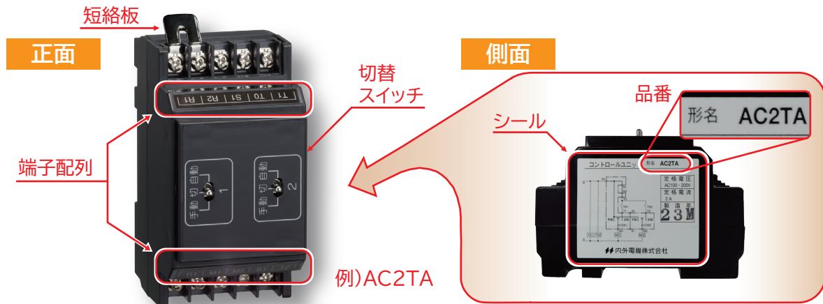
端子配列図
